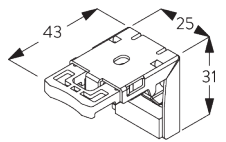
SG 10101 Träger
