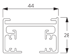
SG 11863 Profil
