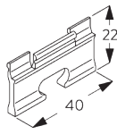
SG 5118 Klammer
