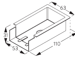
SG 11886 Nutmaske
