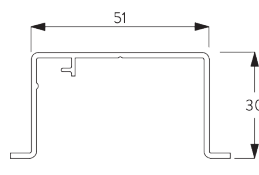
SG 11866 Nutprofil
