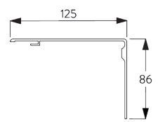
SG 8678 Verdeckter Box Deckel 105x125 mm
