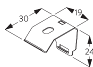
SG 10136 Träger
