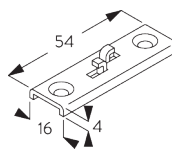
SG 6124 Träger
