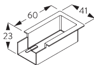
SG 11238 Nutmaske
